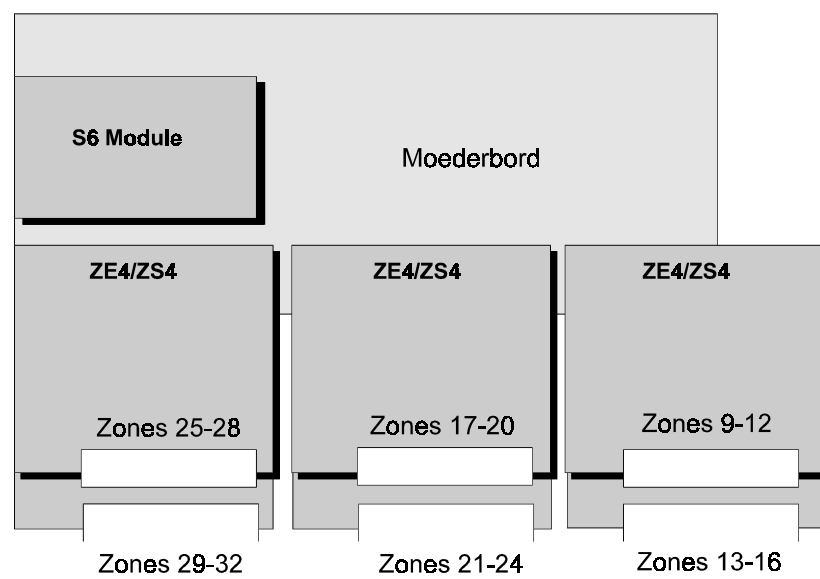
Figuur 5b - Layout van een 32 zone centrale
