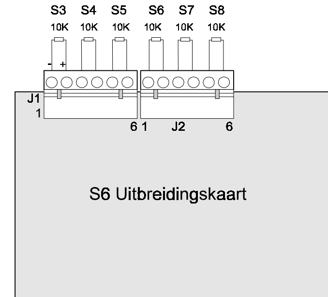
Figuur 13 - Aansluitingsdetails van sirene circuits 3 tot 8
