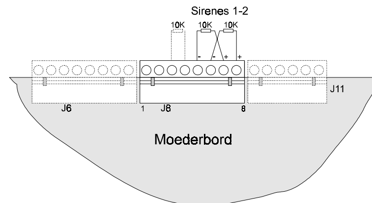
Figuur 12 - Aansluitingsdetails van sirene circuits 1 en 2
