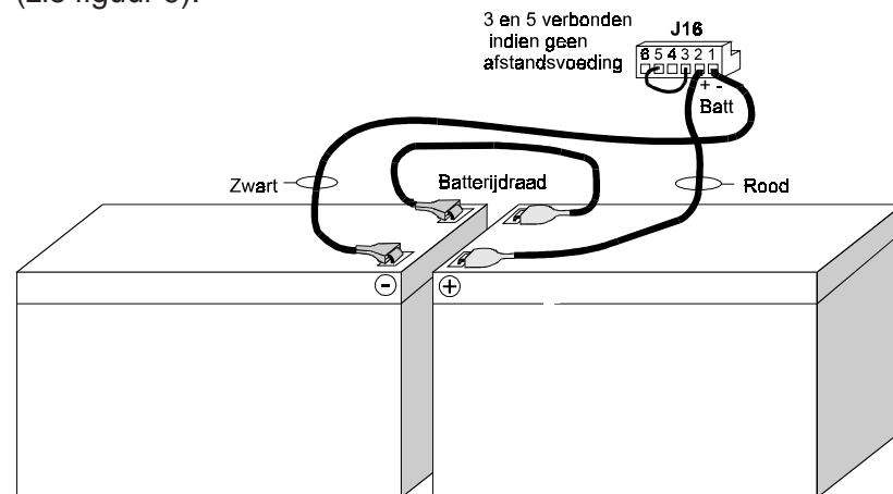
Figuur 9 - Batterij aansluiting
