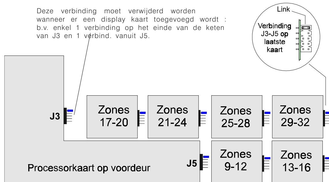
Figuur 4 - Locatie van de display uitbreidingskaart(en)
