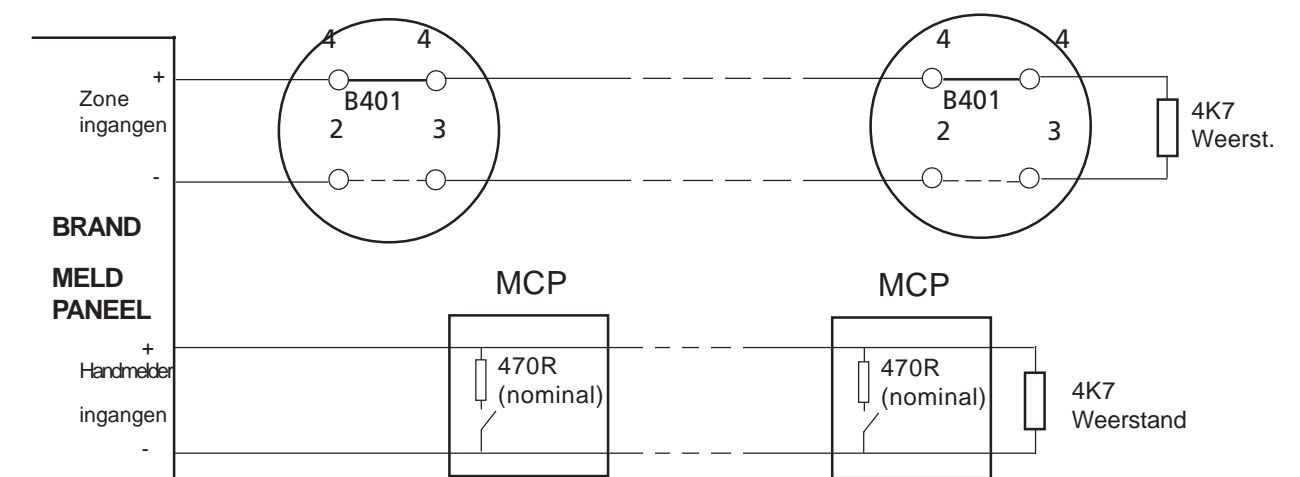
Figuur 6 - Typische sokkel bedrading (B401D)
