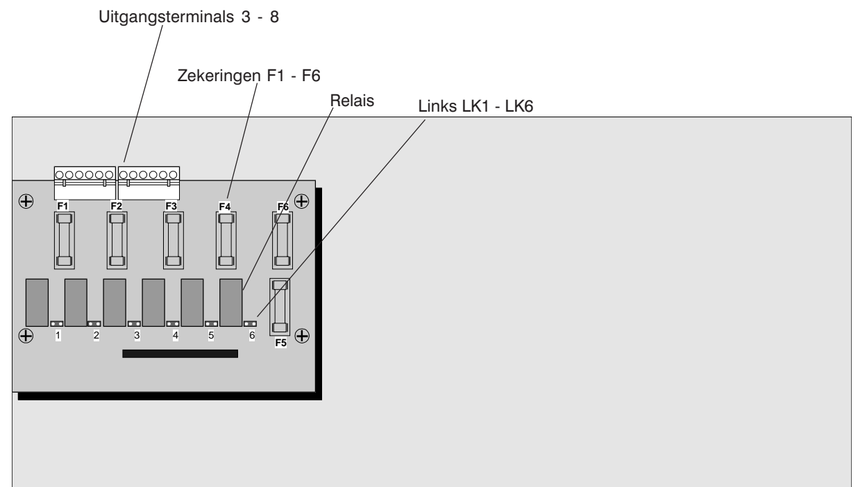
Figuur 3 - S6 Sirene uitbreidingskaart op moederbord
