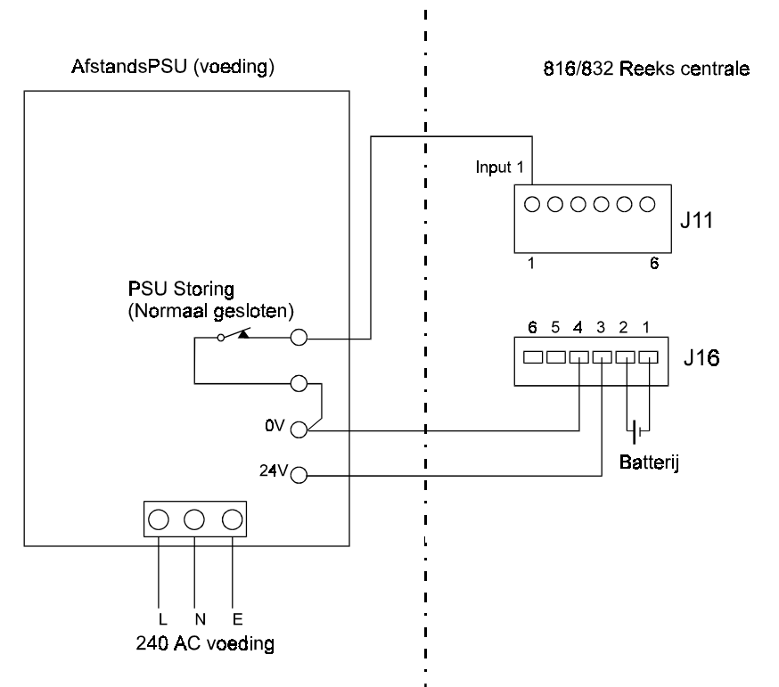
Figuur 19 - Nevenvoeding : Aansluitingsdetails
