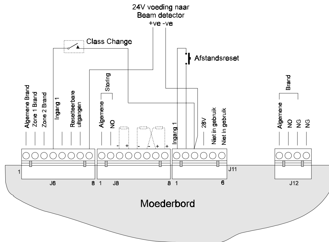
Figuur 17 - Aansluitingsdetails van de Typische Nevenfuncties
