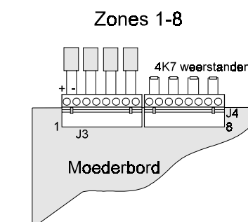
Figuur 10 - Aansluitingsdetails van zones 1 tot 8
