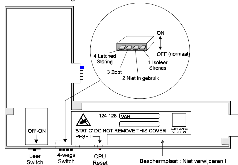
Figuur 8 - Processor kaart met Leer Operatie schakelaar
