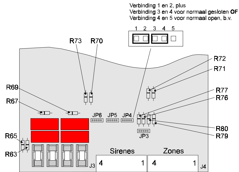
Figuur 18 - Link en zero-ohm weerstand
