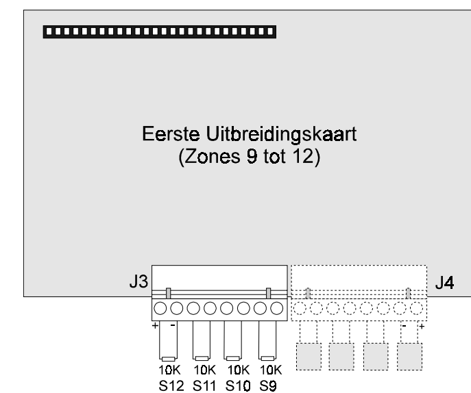
Figuur 14 - Aansluitingsdetails van sirene circuits 9 tot 12
