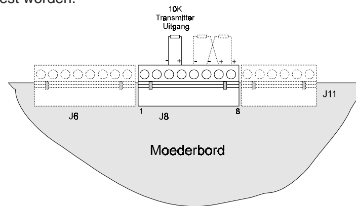
Figuur 15 - Aansluitingsgegevens voor de Transmitter uitgang
