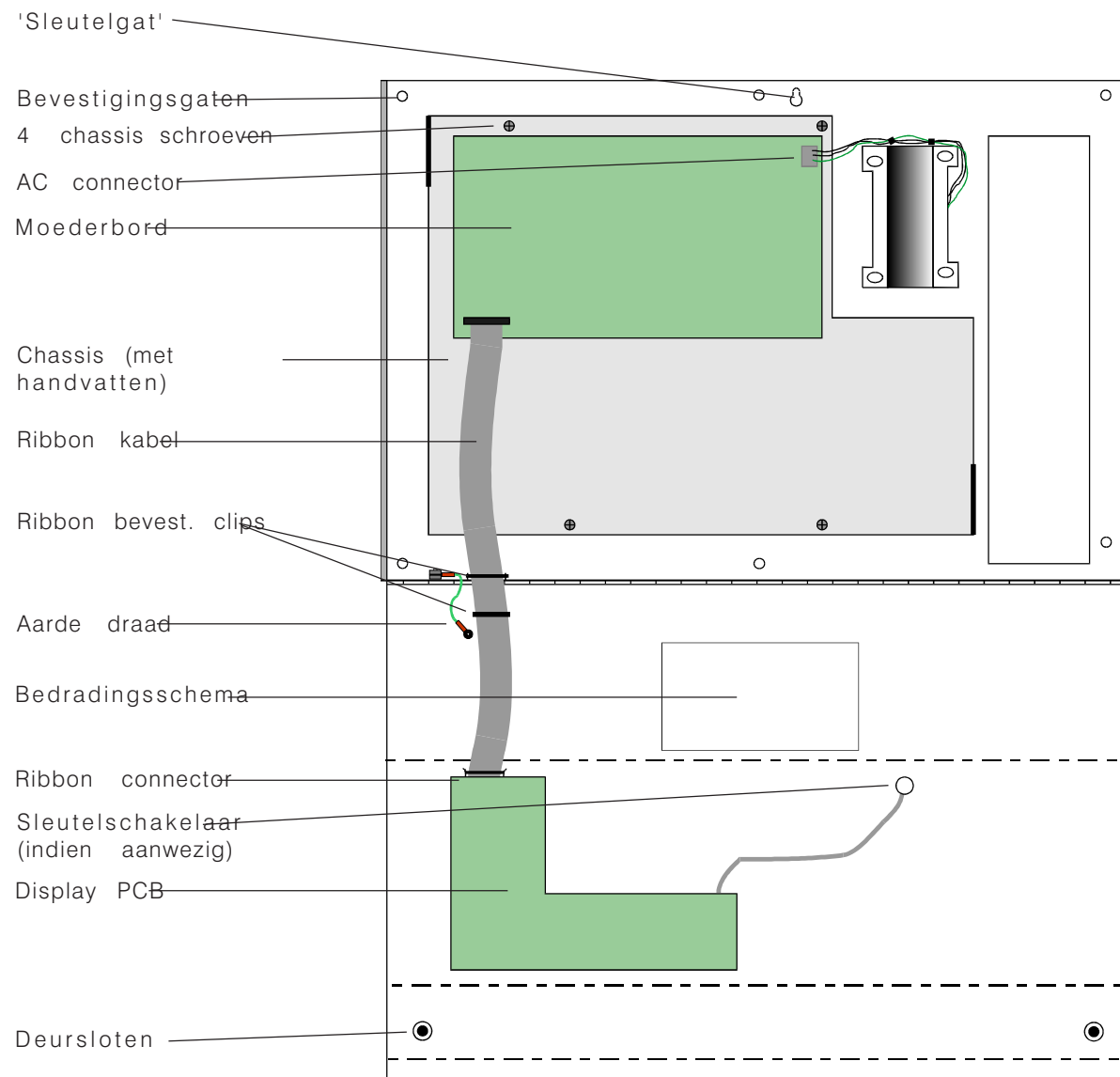
Figuur 2 - Interne layout (32 zone) met 8 zones gemonteerd.
