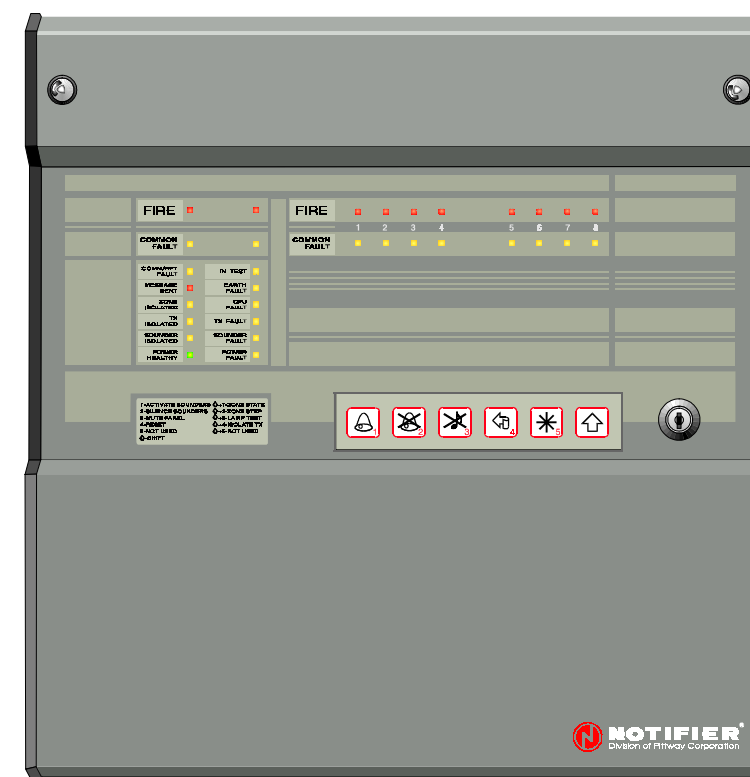
Figuur 1 : 8-zone brandmeldcentrale zonder veiligheidsdeur
