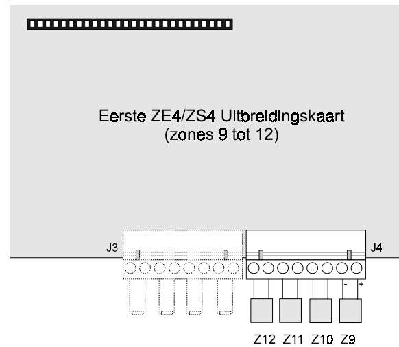
Figuur 11 - Aansluitingsdetails van zones 9 tot 12
