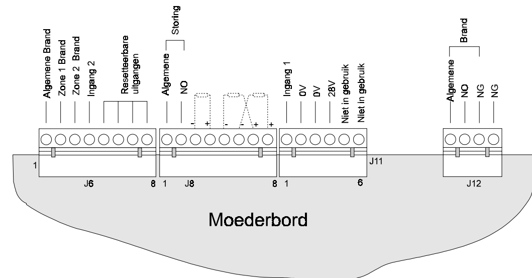
Figuur 16 - Aansluitingsdetails van Neven in en -uitgangen
